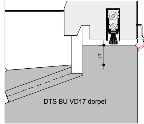
Deurvak (D) Binnendraaiend
