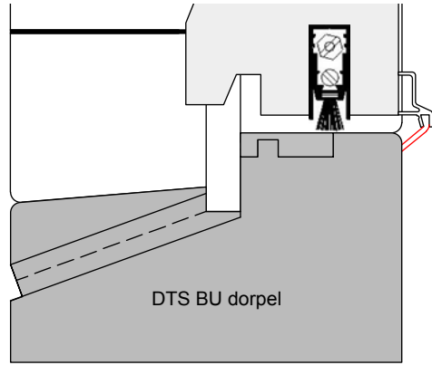
Deurvak (D) Binnendraaiend BUV lat 7x27 mm
