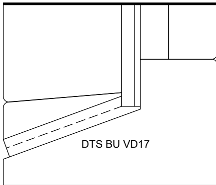
Doorsnede
