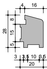
KAI Binnenlat
