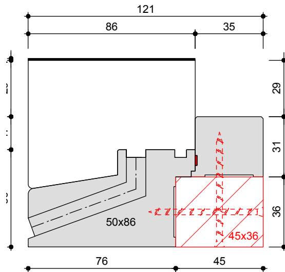
Hybride deurvak DTS BU KAI Passief kozijnmaat 67 x 121
