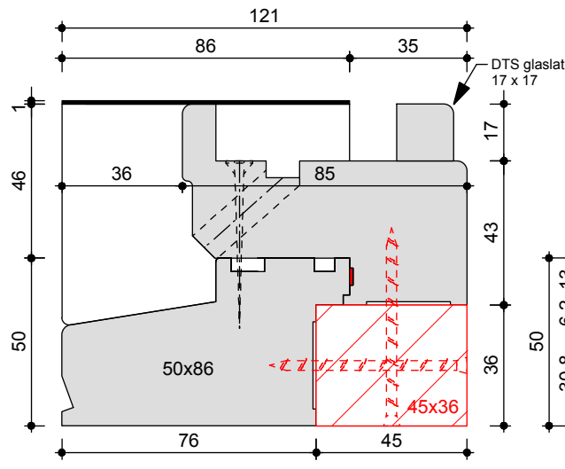
Hybride glasvak DTS BU KAI Passief kozijnmaat 67 x 121
