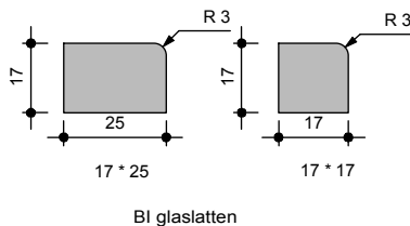
BI glaslatten
