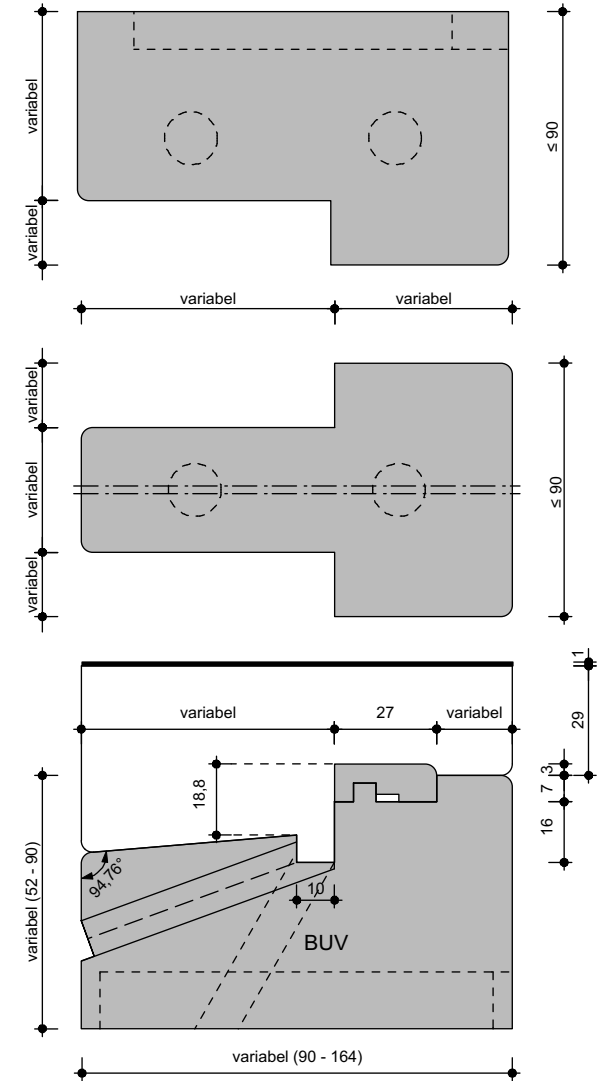
BUV --> kozijnen met een buitensponning en een kaderdichting
