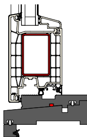
BUITEN ADAPTER
