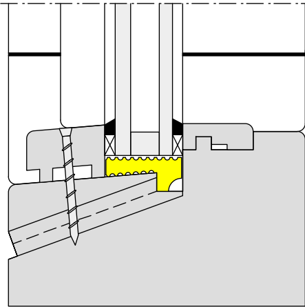
Glasvak (G)
