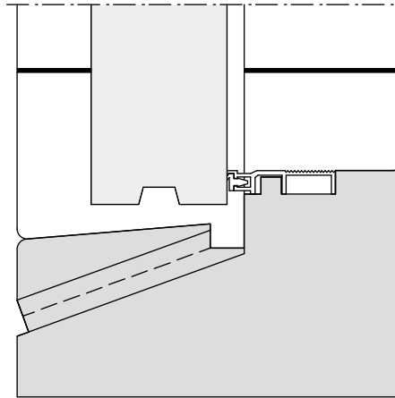
Deurvak (D)
