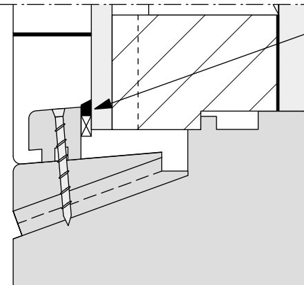
Glas-Paneelvak (GP)
