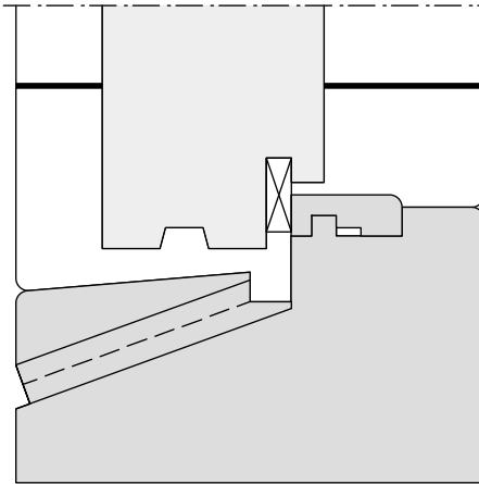
Kaderdeurvak (K)
